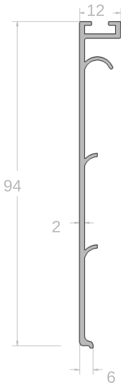
INNER COVER PROFILE UNUTRAŠNJI POKLOPNI PROFIL
