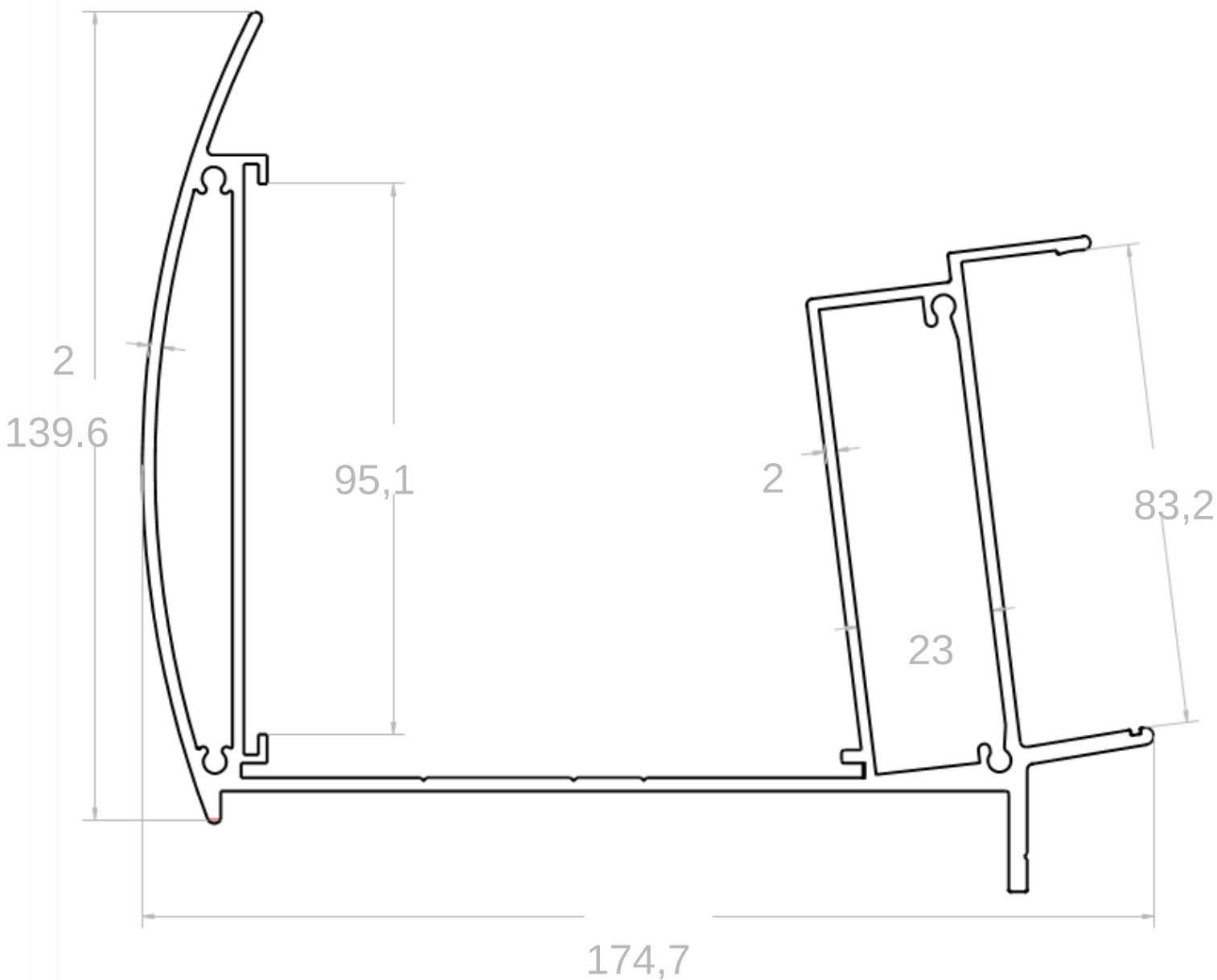
GUTTER PROFILE OLUČNI PROFIL
