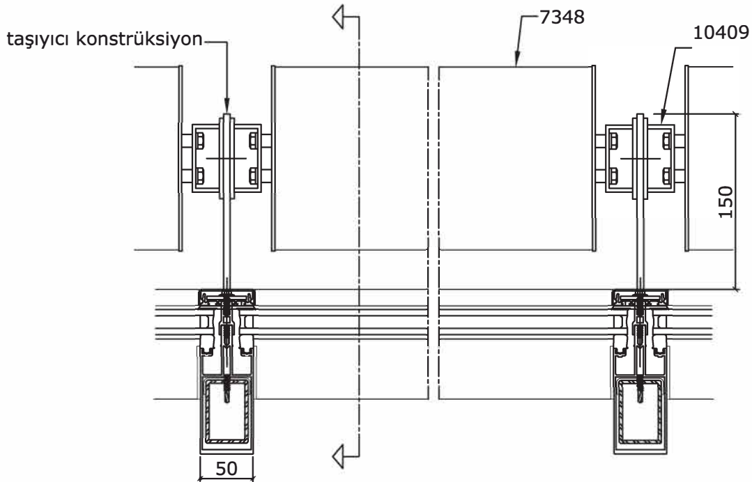
KESİT
