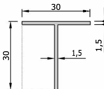
705 0,245 kg/m T Guide Profile
