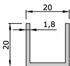
843 0,285 kg/m U Guide Profile
