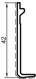
257 Eko osigurači stakla 0,245 kg/m ( Siva mat eloksaža )
