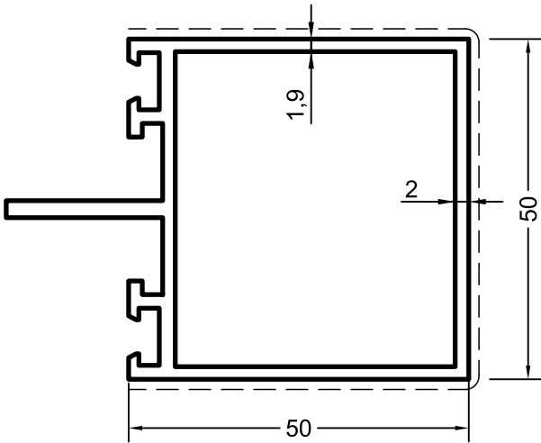
211 Horizontala za silikonske fuge 1,220 kg/m J_x = 14,46 \text{ cm}^4 J_y = 19,15 \text{ cm}^4
