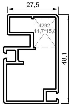
292 Eko krilo 0,730 kg/m
