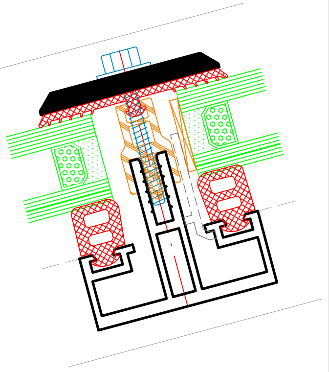
Poklopac krovni
