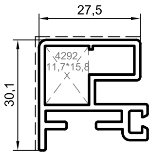
254 Eko krilo 0,630 kg/m
