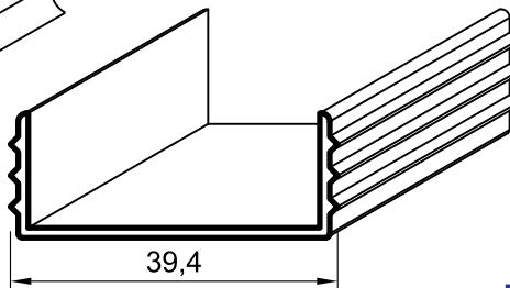
242 ( Rezano na 36 mm ) Dilatacioni poklopac 0,230 kg/m
