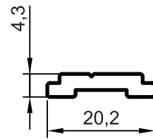
4293 Pogonska letva 0,180 kg/m
