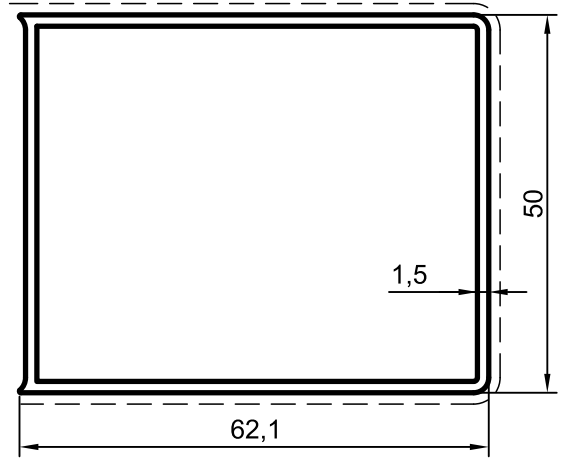
270 Dopuna horizontale 0,885 kg/m J_x = 13,39 \text{ cm}^4 J_y = 18,34 \text{ cm}^4
