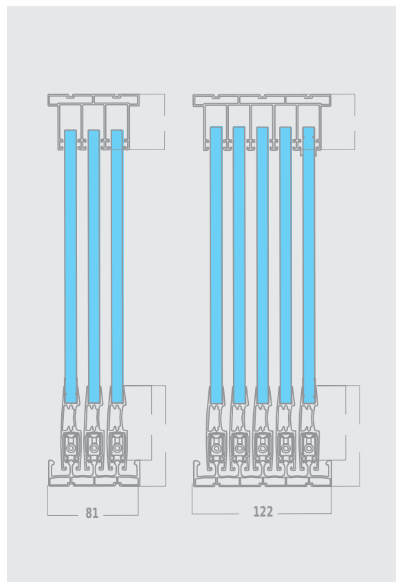
DONJA ŠINA (5 KANALA) BOTTOM RAIL ( 5 )
